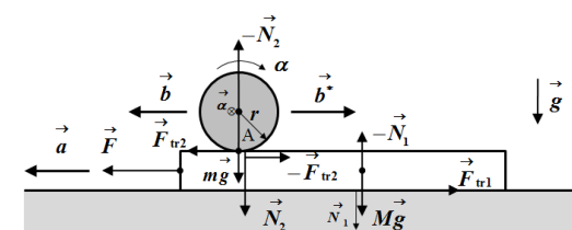
Слика 2. Инерцијални систем
